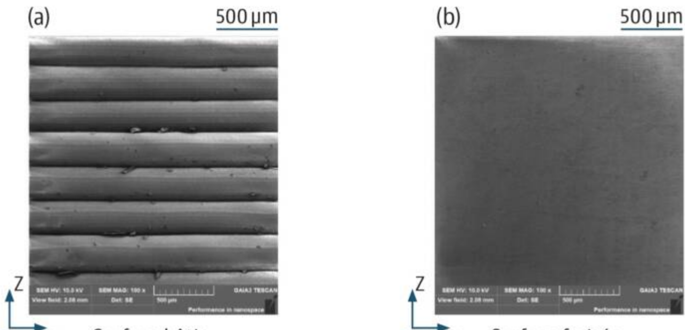
Figure 8. Pièce hybride additive-soustractive en polymère
